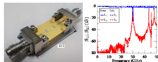
(b) 金導体(実測値) ハット30GHz帯フィルタ
