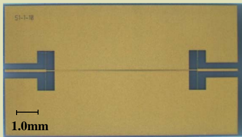
(a) 試作した \lambda/2 共振器
