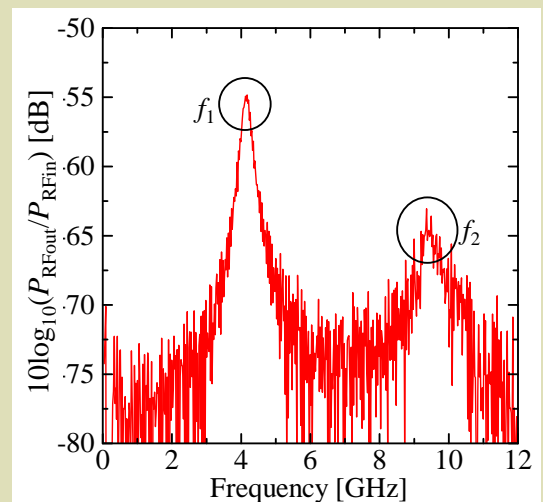
(b) 周波数応答の測定結果
