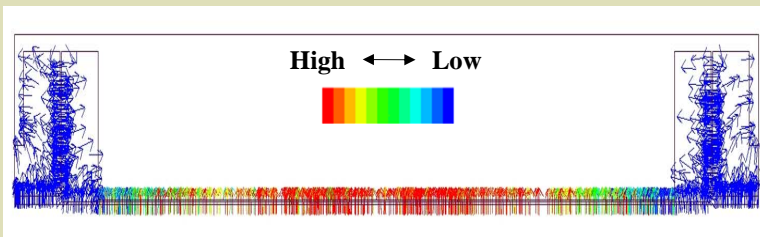
(c) 電界分布(@ f_1 )
