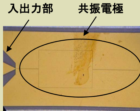
(b) 試作した共振電極
