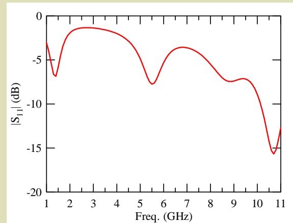
(c) |S_{11}| の計算結果
