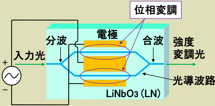
(a) MZ型光変調器の基本構造
