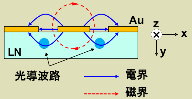
(b) 電磁界分布 (断面図)
