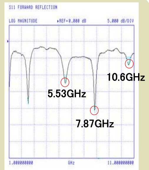
(c) |S_{11}| の測定結果
