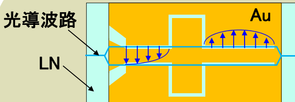
(a) 電界分布の設計仕様
